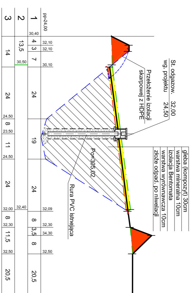
Przekroj 0+24,5
